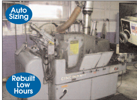
CINCINNATI # OM CENTERLESS GRINDER
