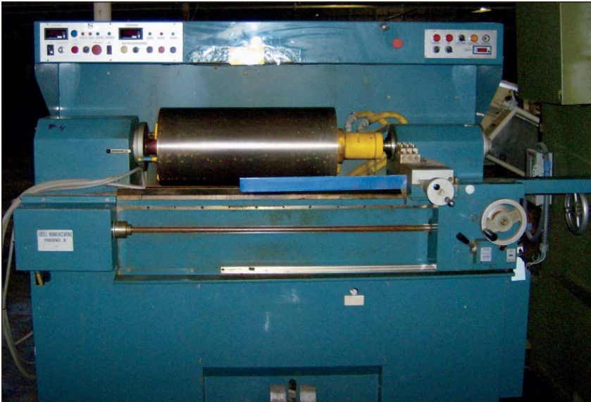
Fioa Ice Lathe, 27.5" Barrel
